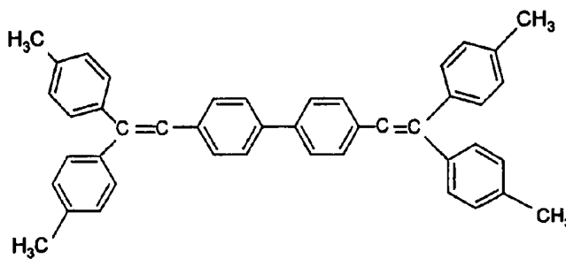
DTVb1
