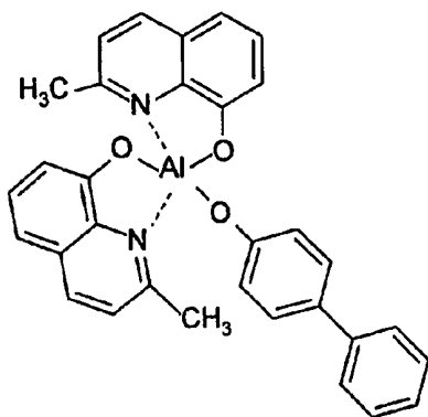
BAlq1
