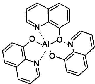
Alq
