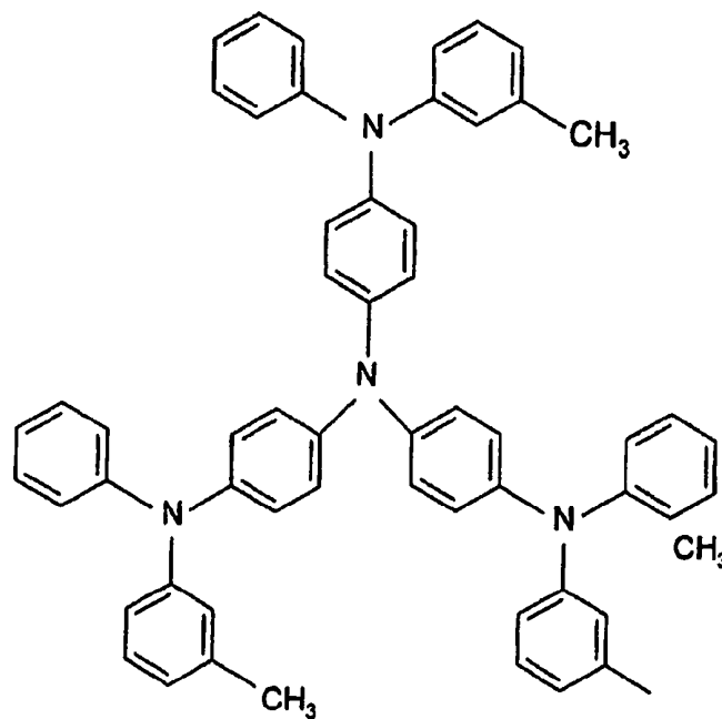
mTADATA
